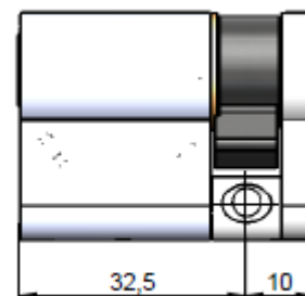
Cylindre simple
